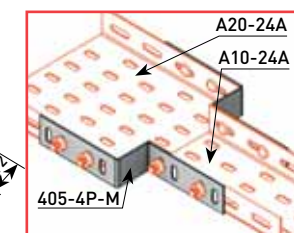
405-4P-M — Пример соединения
