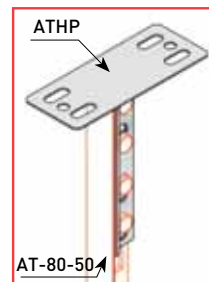
АТНР-В — Пример соединения
