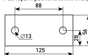
Размеры и расположения отверстий
