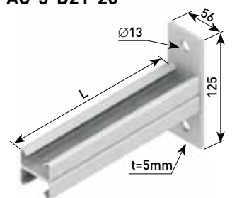
Размеры и расположения отверстий
