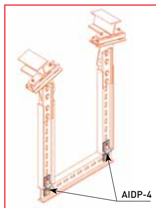
АІДР-4 — Пример соединения
