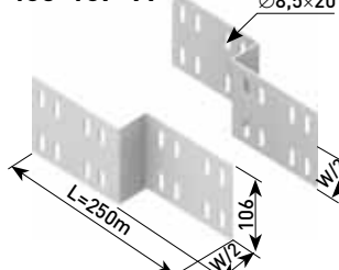
405-10P-M — Пример соединения
