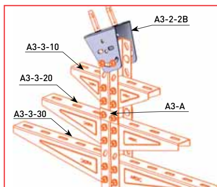
A3-2-2B — Пример соединения
