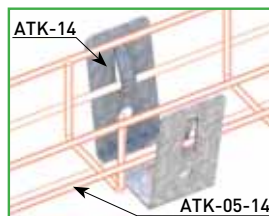
ATK-14 — Пример соединения
