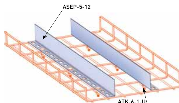
ASEP-50-10 — Пример соединения с АТК-6-1-U
