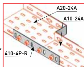
410-4P-R — Пример соединения
