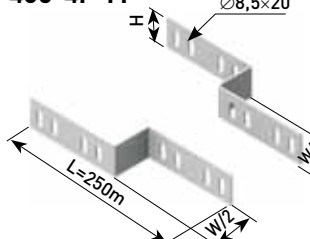
405-4P-M — Пример соединения
