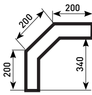
720-10A— Пример соединения
