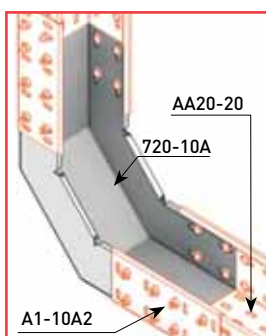
720-10A— Пример соединения
