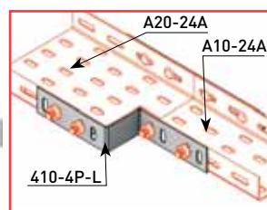
410-4P-L — Пример соединения
