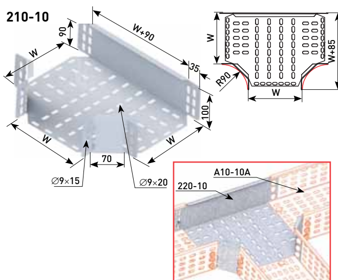
220-10 – Пример соединения
