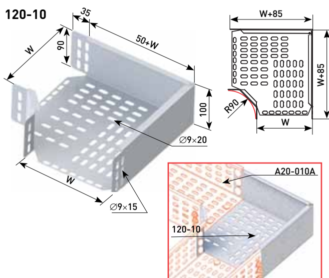
120-10 – Пример соединения
