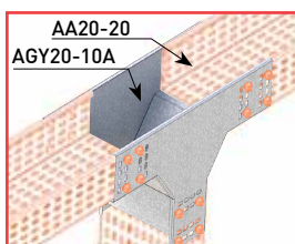
AGY20-10A— Пример соединения
