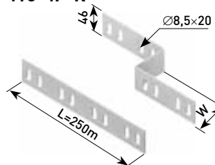
410-4P-R — Пример соединения
