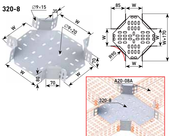
320-8 — Пример соединения
