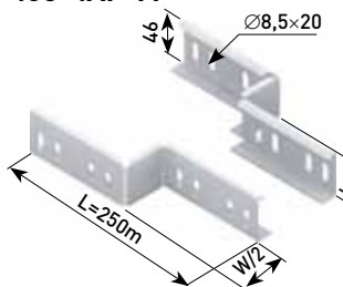
405-4AP-M — Пример соединения
