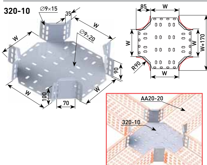
320-10 — Пример соединения
