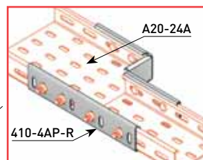
410-4AP-R — Пример соединения
