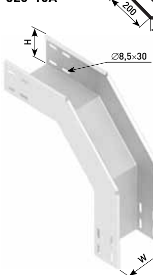
820-10A— Пример соединения
