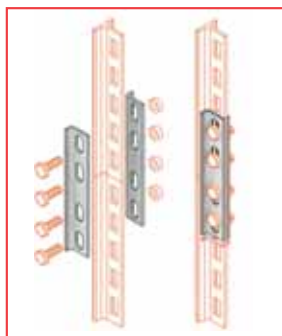
АТНР-1 — Пример соединения
