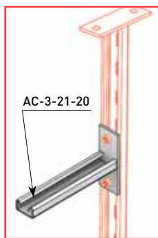
AC-3-21-20 — Пример соединения
