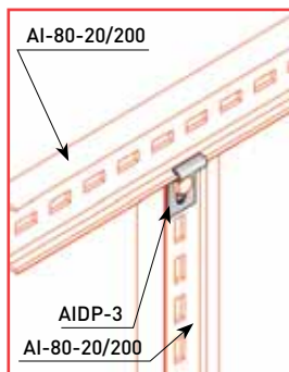
АІДР-3 — Пример соединения
