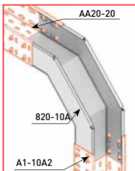
820-10A— Пример соединения
