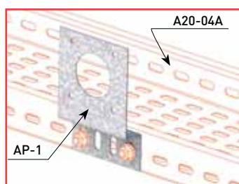
AP-1 — Пример соединения
