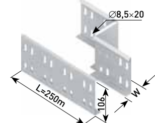
410-10AP-R — Пример соединения
