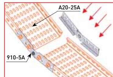
901-5A— Пример соединения
