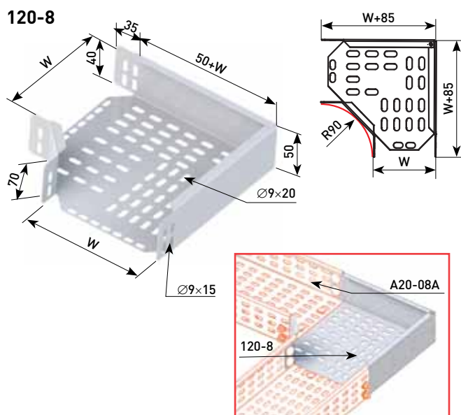
120-8 — Пример соединения
