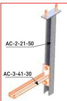
AC-2-21-50 — Пример соединения
