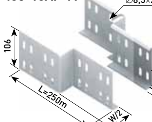
405-10AP-M — Пример соединения
