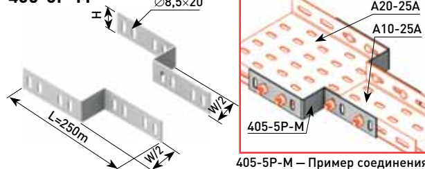
405-5P-M — Пример соединения
