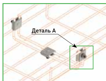
АТК-6-2 – Пример соединения
