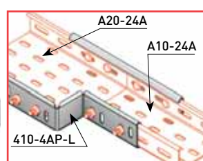
410-4AP-L — Пример соединения
