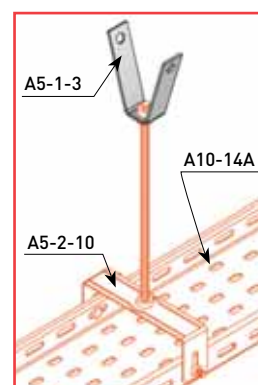
A5-1-3 — Пример соединения
