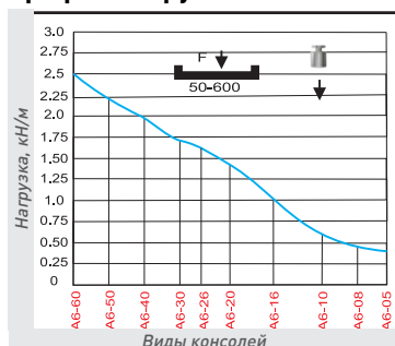
A6-20 — Применение консолей
