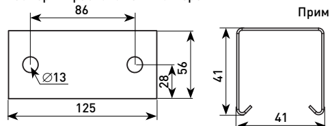
Размеры и расположения отверстий
