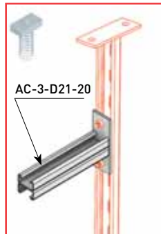
AC-3-D21-20 — Пример соединения
