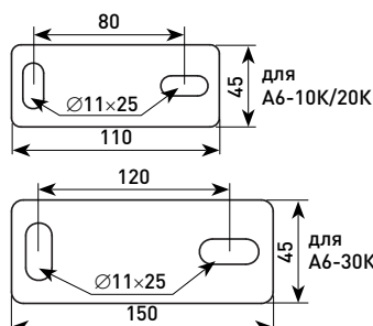
A6-20K — Применение консолей
