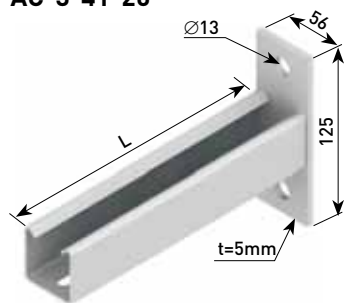
Размеры и расположения отверстий
