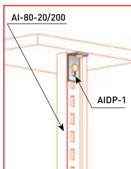
АІДР-1 — Пример соединения
