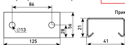
Размеры и расположения отверстий
