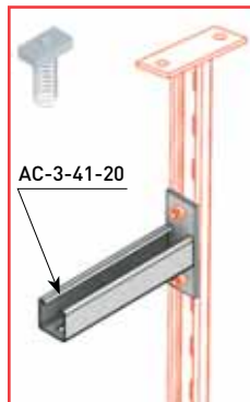
AC-3-41-20 — Пример соединения
