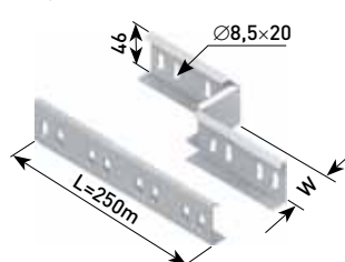
410-4AP-R — Пример соединения
