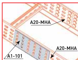
A1-101 – Пример соединения
