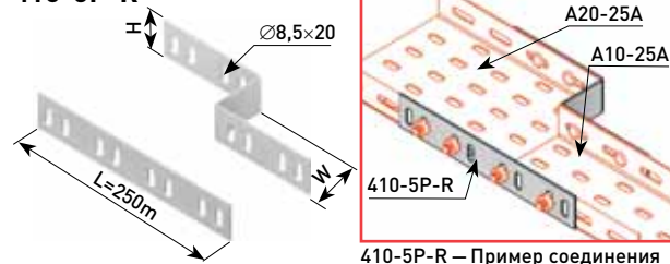
410-5P-R — Пример соединения
