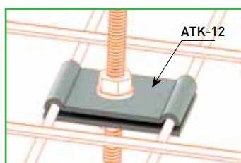
АТК-12 — Пример соединения
