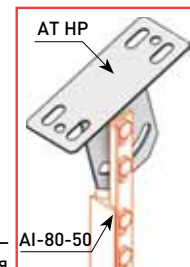
АТНР — Пример соединения
