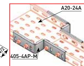
405-4AP-M — Пример соединения
